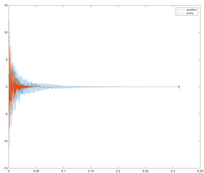
Figura 61 – Comparação entre h(t) analítico e reconstrução por Prony — Davi
